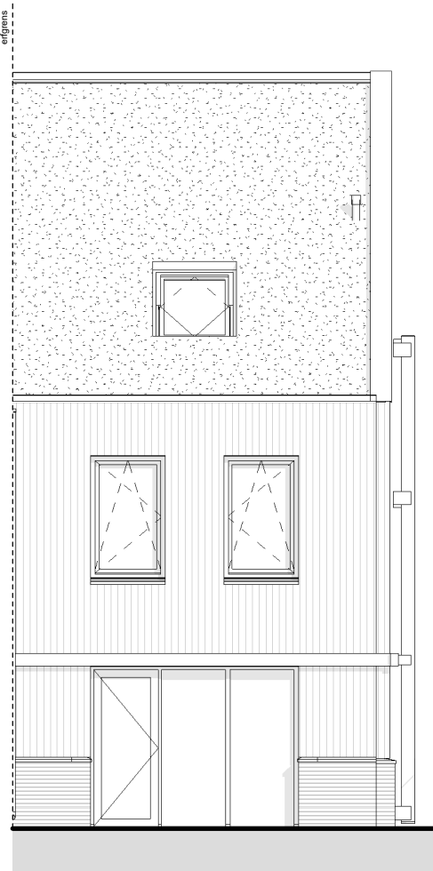
achtergevel (noord)
